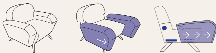
Smontaggio braccioli / Dismantling armrests / Démontage accoudoirs / Demontage der Armlehnen
